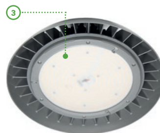
PC-Linsen für Abstrahlwinkel 90D oder 60D
